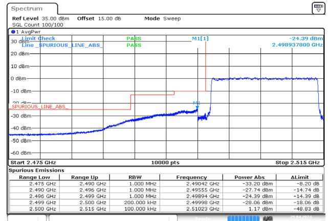
15MHz_Low_QPSK_75@0 -24.39dBm
