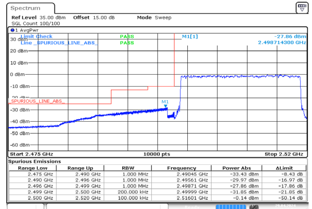
20MHz_Low_QPSK_100@0 -27.86dBm
