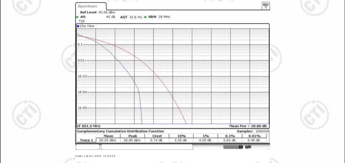
Band26-10MHz-QPSK-26865-1RB#0
