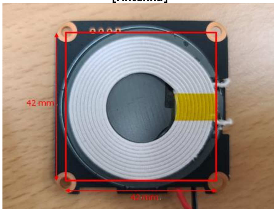
[Antenna]
