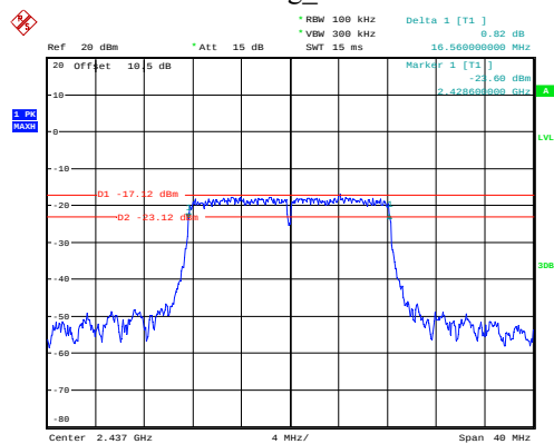
802.11g_2437MHz
