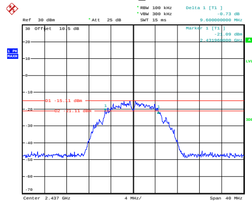
802.11b_2437MHz
