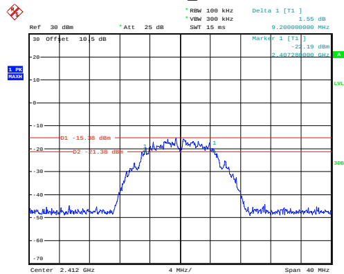
802.11b_2412MHz
