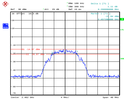
802.11b_2462MHz
