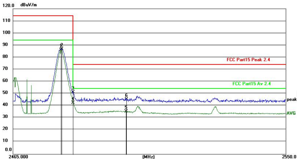
2480MHz Horizontal
