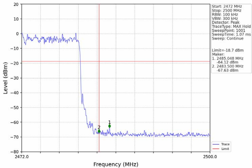
Pi/4QPSK_2DH5_HOPP_Ant1_NTNV
