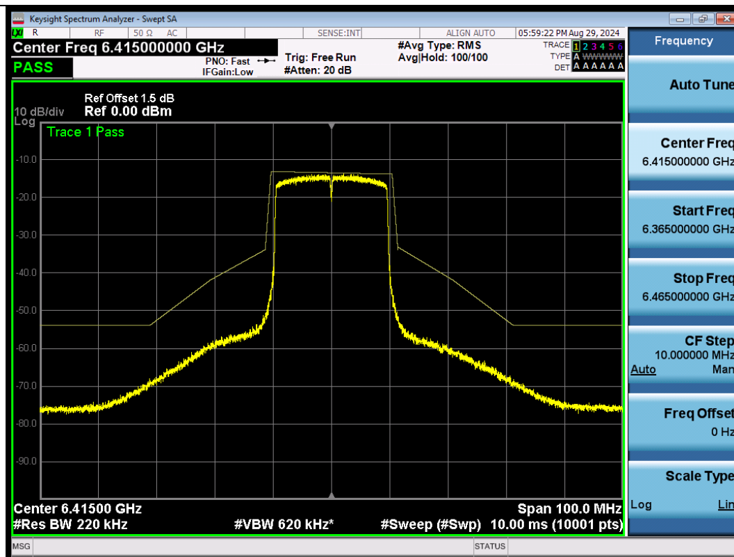
NTNV-11AX20SISO-Ant1-6415-PASS
