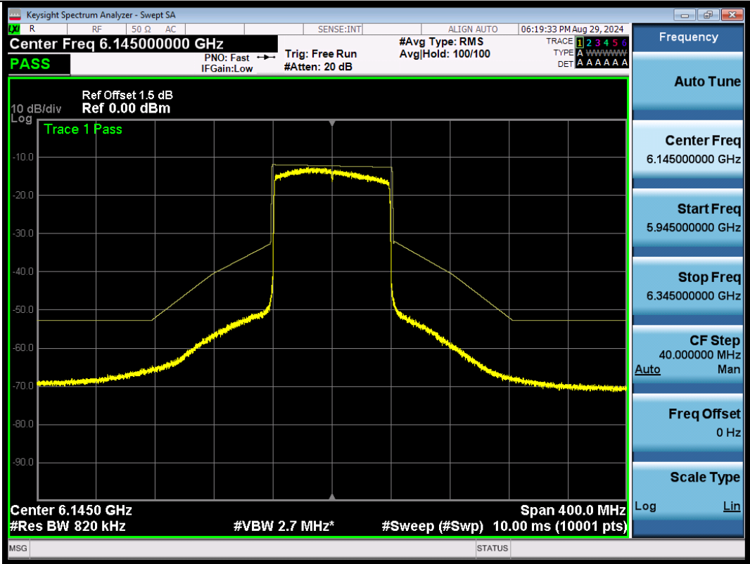
NTNV-11AX80SISO-Ant1-6145-PASS
