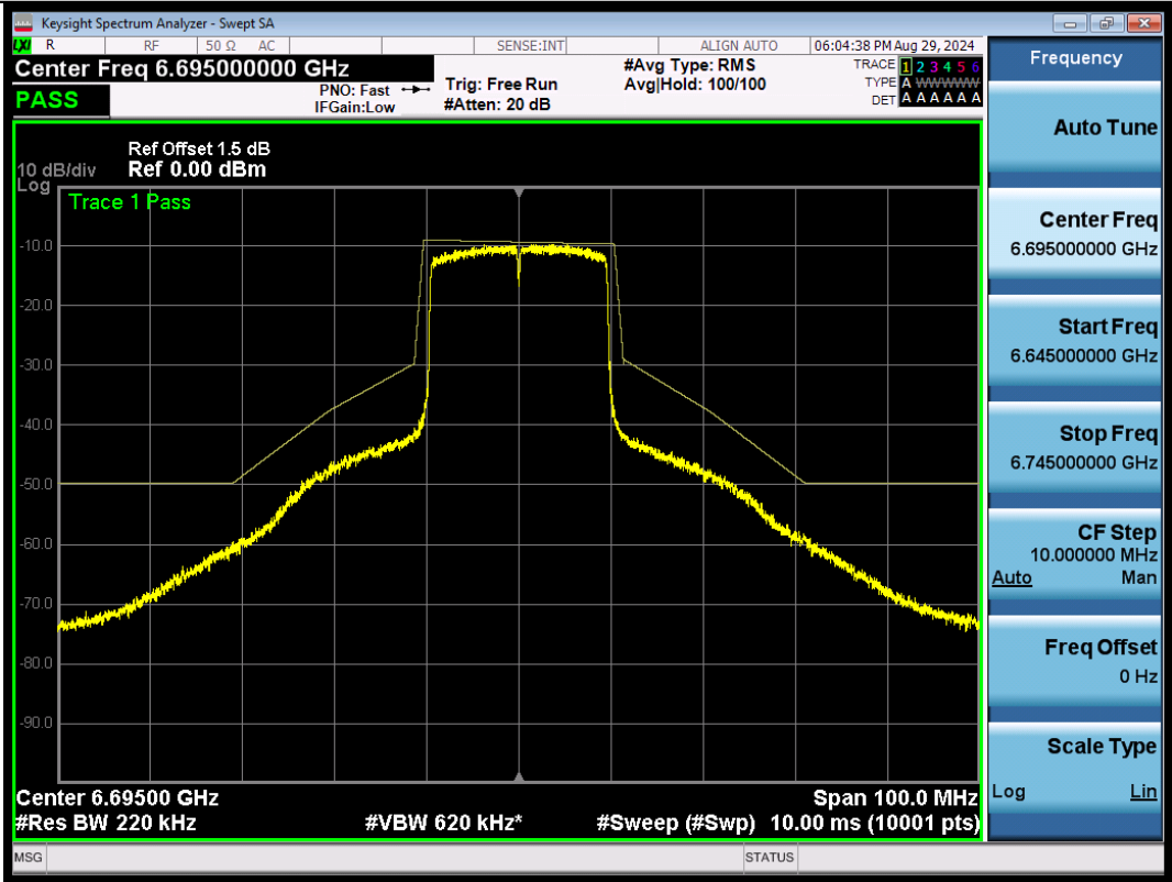
NTNV-11AX20SISO-Ant1-6695-PASS
