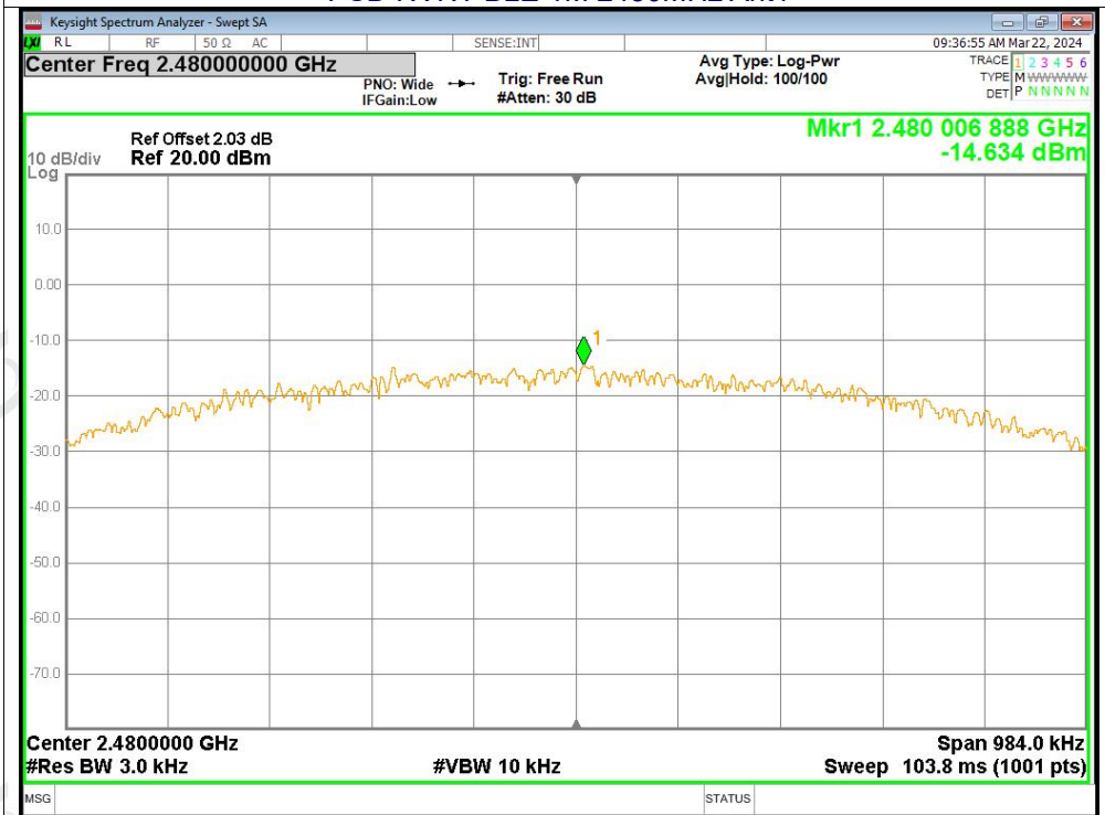
PSD NVNT BLE 1M 2480MHz Ant1
