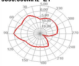
5850.000MHz E1
