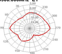
5500.000MHz E1
