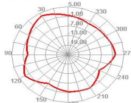
2500.000MHz E2
