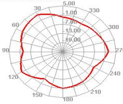
2450.000MHz H
