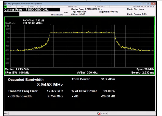
Band 4 10MHz/1715.0/Low QPSK 50@0
