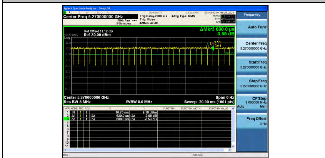
11AC40MIMO_Ant1_5270
