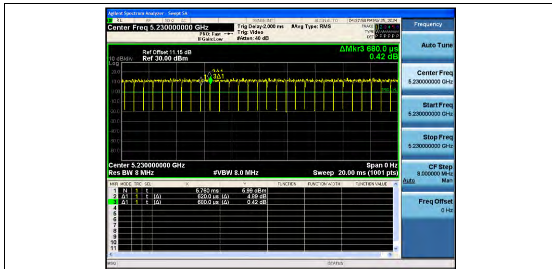
11AC40MIMO_Ant2_5230
