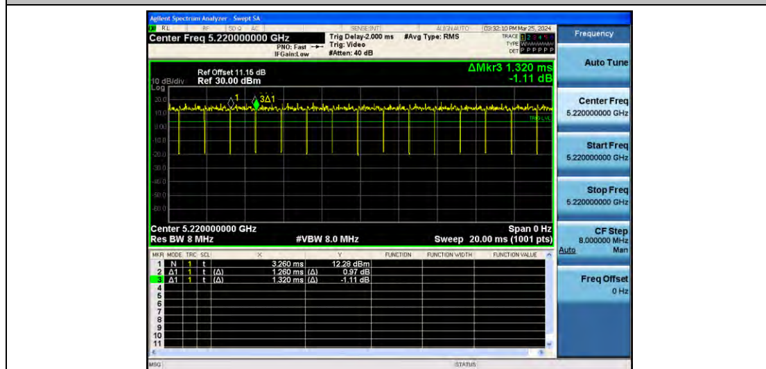
11AC20MIMO_Ant2_5220
