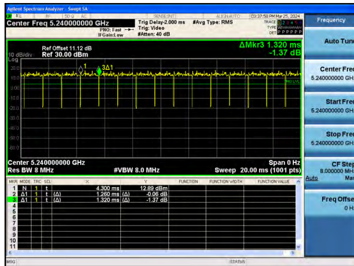
11AC20MIMO_Ant2_5240
