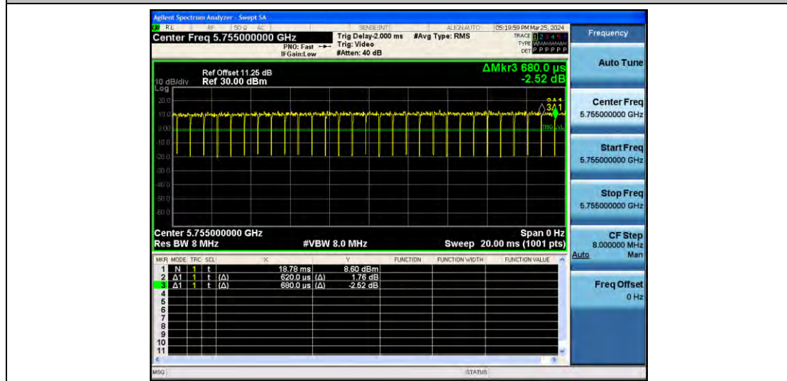
11AC40MIMO_Ant1_5755
