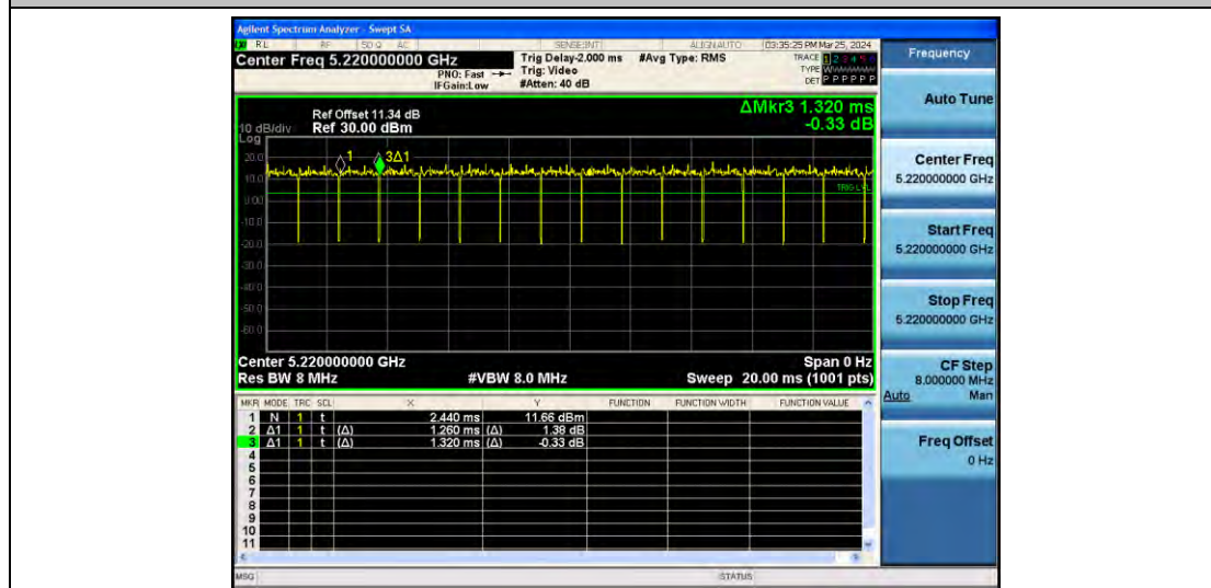
11AC20MIMO_Ant2_5220
