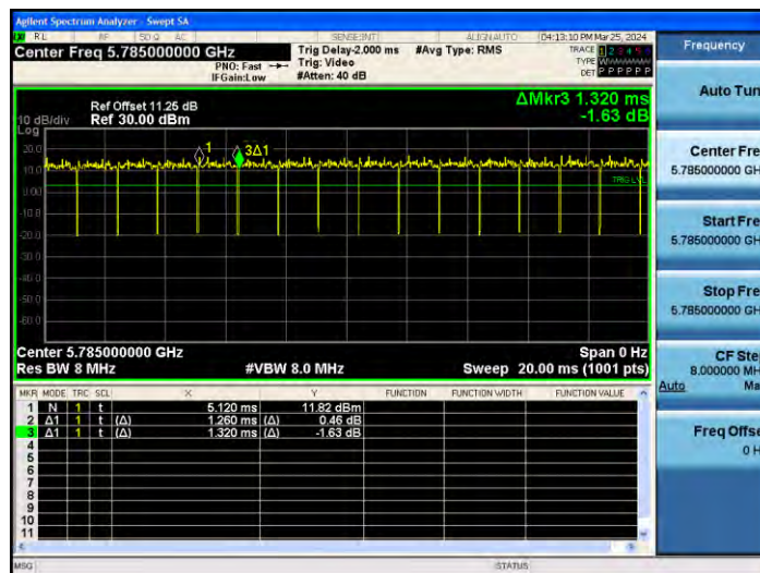
11AC20MIMO_Ant2_5785
