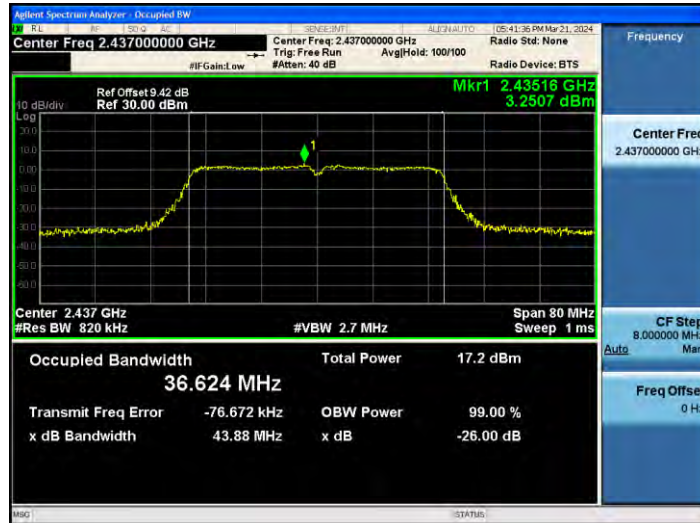
11N40MIMO_Ant2_2437
