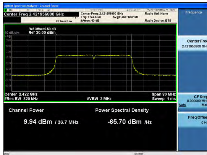
11N40MIMO_Ant2_2422
