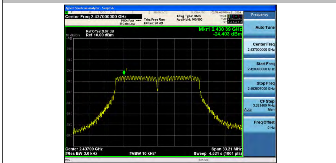
11G_Ant2_2437
