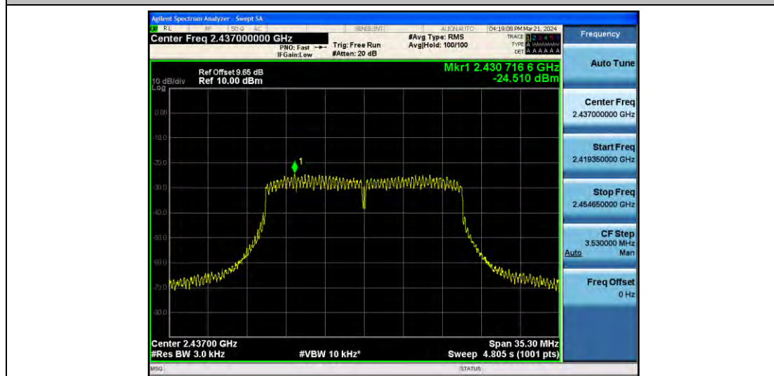
11N20MIMO_Ant1_2437
