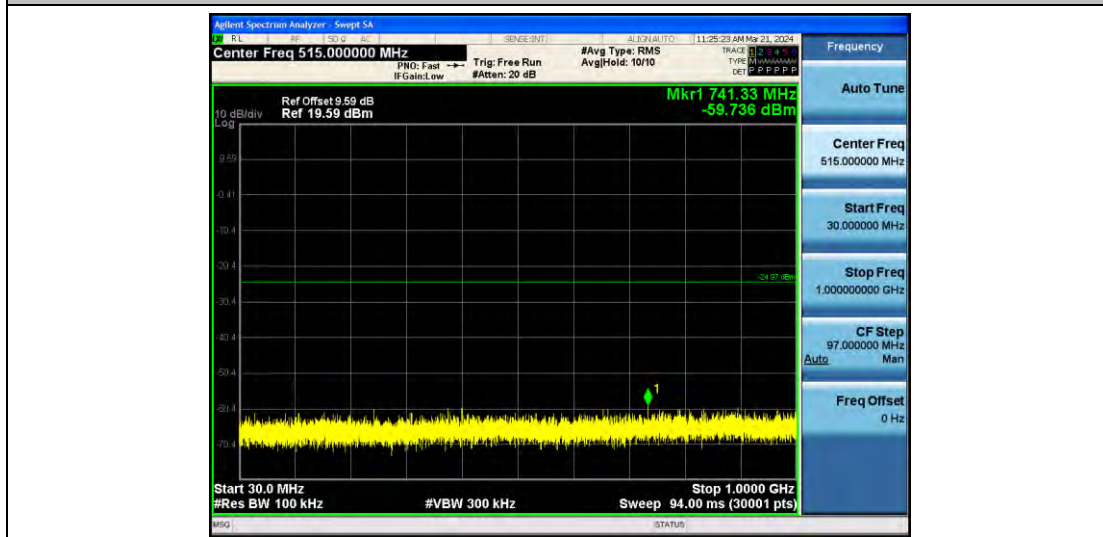
11B_Ant2_2412_30~1000
