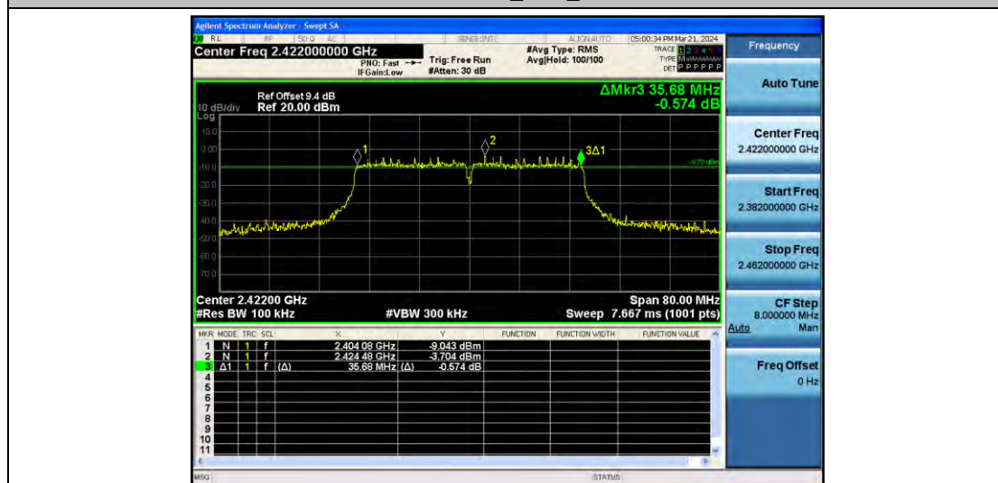
11N40MIMO_Ant2_2422
