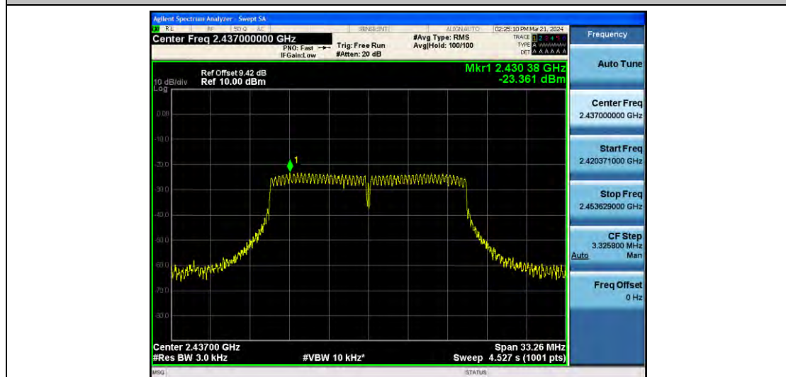
11G_Ant2_2437
