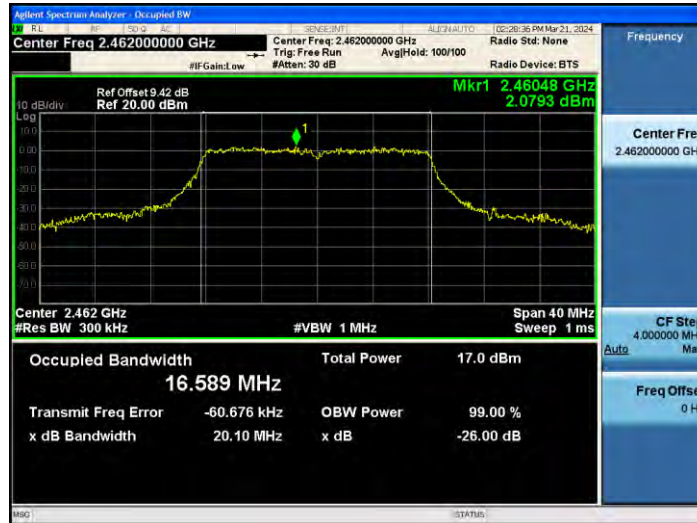
11G_Ant2_2462
