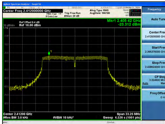
11G_Ant2_2412
