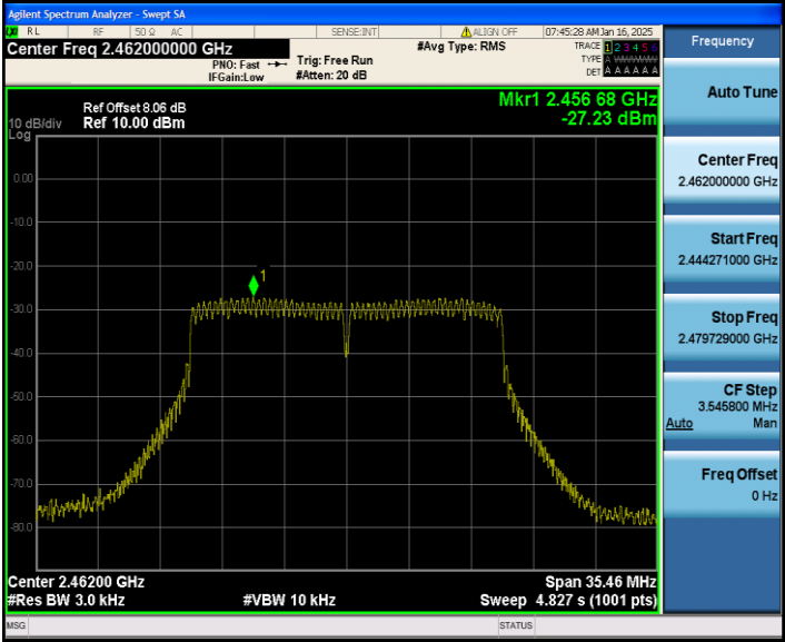
11N20MIMO_Ant2_2462
