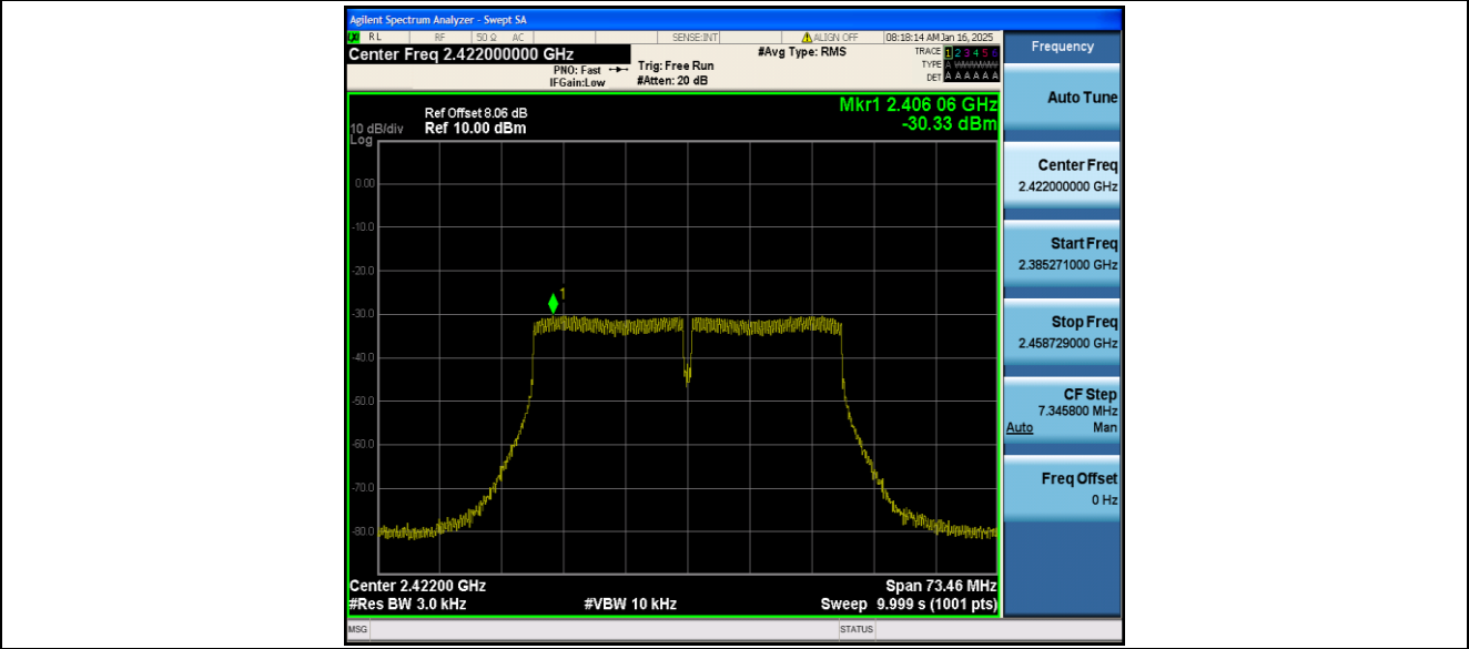
11N40MIMO_Ant2_2422
