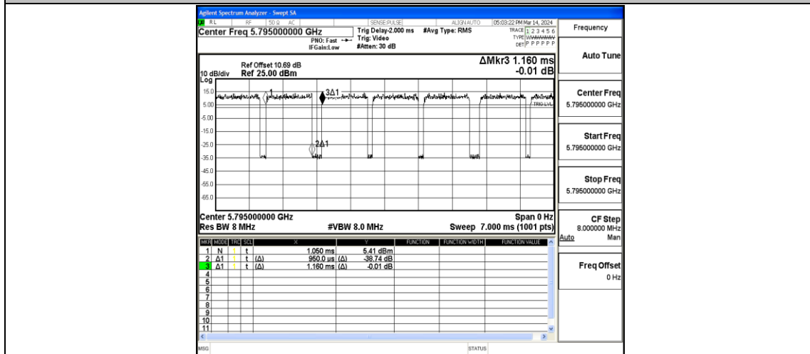
NTNV-11N40MIMO-Ant1-5795
