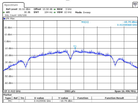
802.11b_2412MHz
