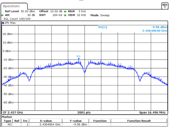
802.11b_2437MHz
