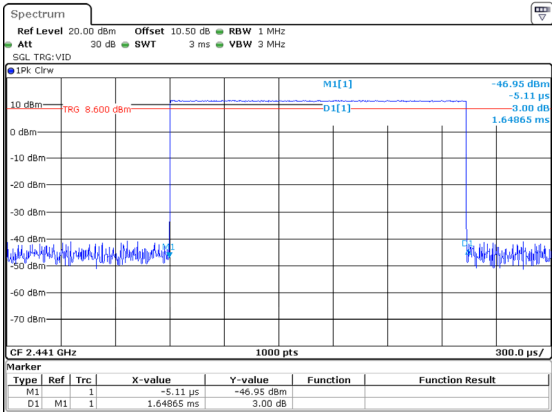
DH3_Hopping 1.649ms
