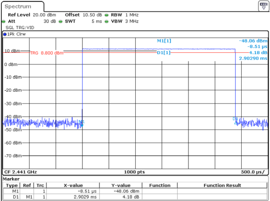
DH5_Hopping 2.903ms
