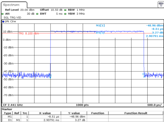
2DH5_Hopping 2.908ms
