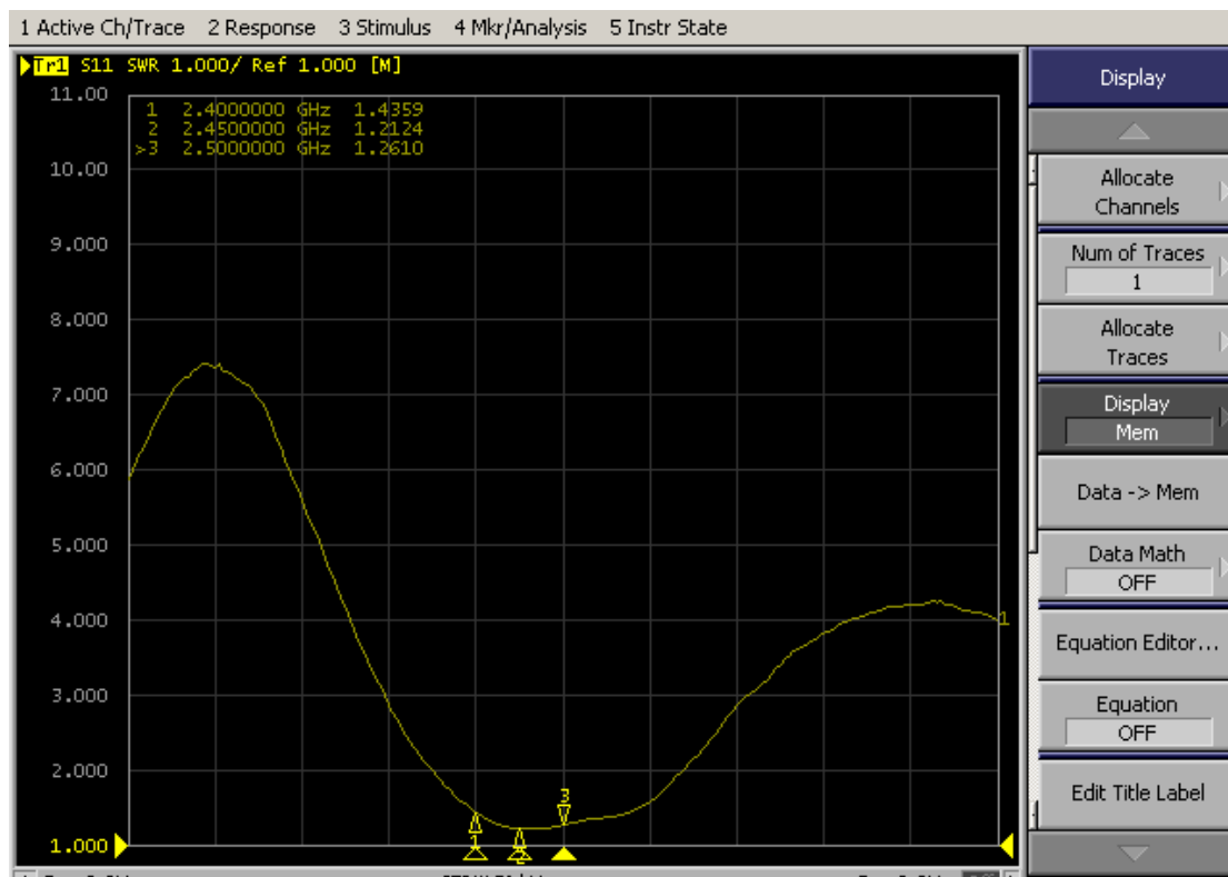
图四、SWR 波形图
