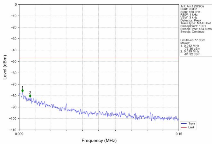
802.11g_LCH_2412MHz_Ant1 (SISO)_NTNV
