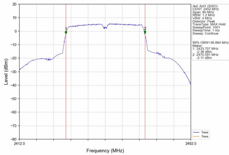
802.11n(HT40) HCH 2452MHz Ant1 (SISO) NTNV
