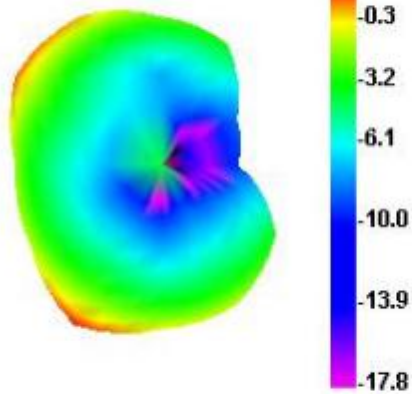
2430.000MHz
