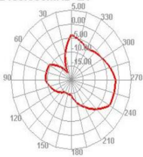
2430.000MHz E1
