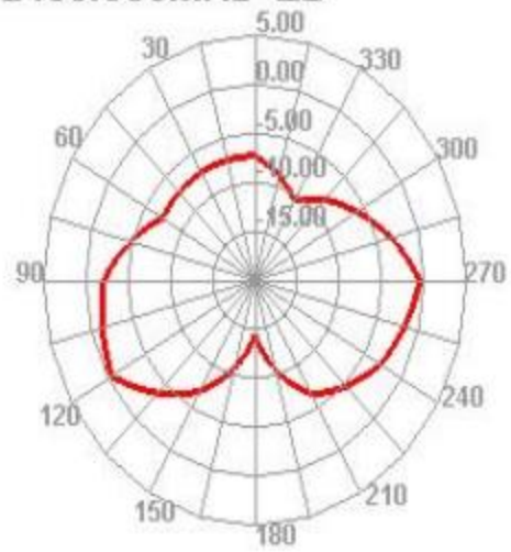
2430.000MHz E2
