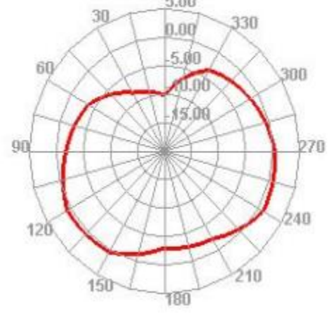
2470.000MHz H
