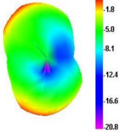
2490.000MHz
