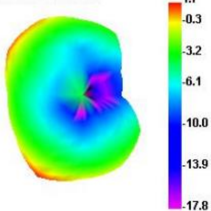
2430.000MHz
