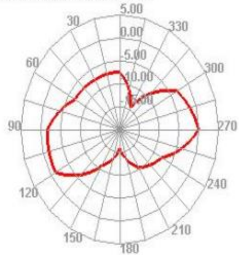
2490.000MHz E2
