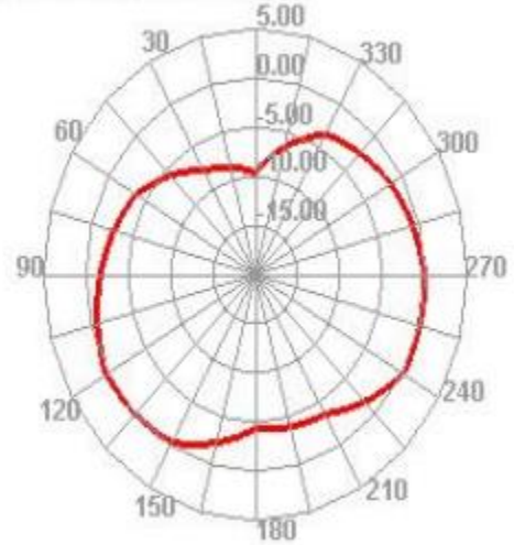
2490.000MHz H
