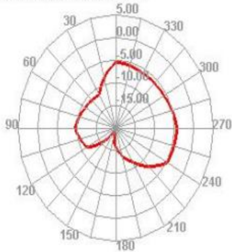
2490.000MHz E1
