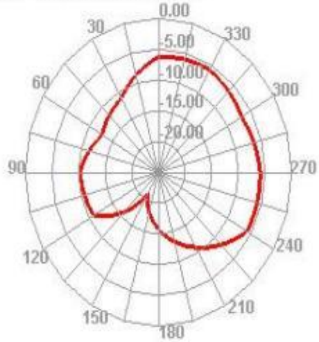
2500.000MHz E1
