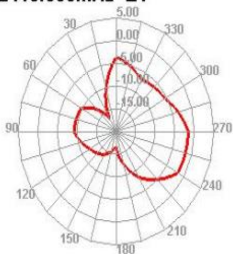
2410.000MHz E1
