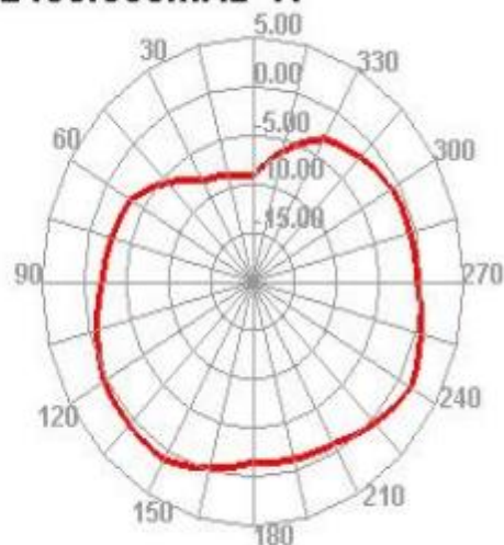
2430.000MHz H
