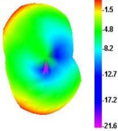
2480.000MHz
