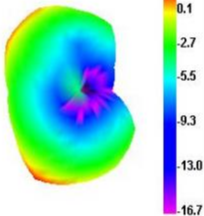
2440.000MHz
