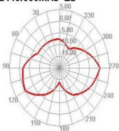
2440.000MHz E2
