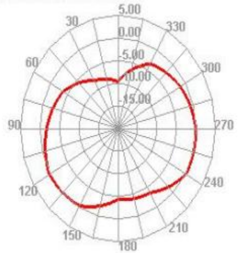
2490.000MHz H
