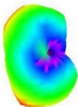
2440.000MHz
