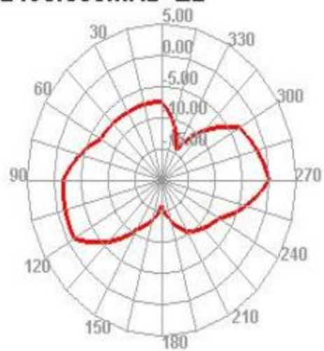
2490.000MHz E2
