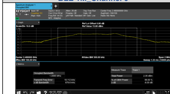
BLE 1M_Channel 39
