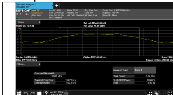
BLE 1M_Channel 0
