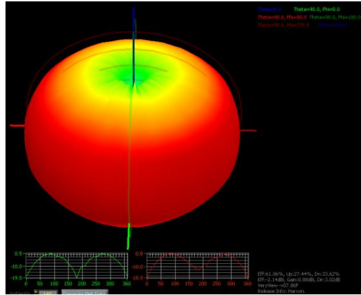
930MHZ
