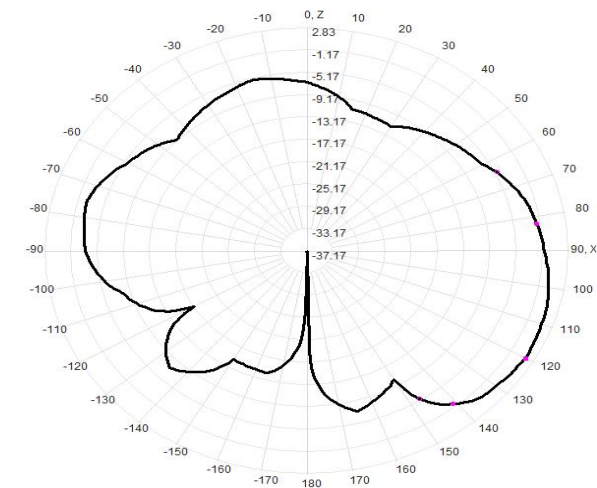
870.0MHz Total(E1-XZ)
