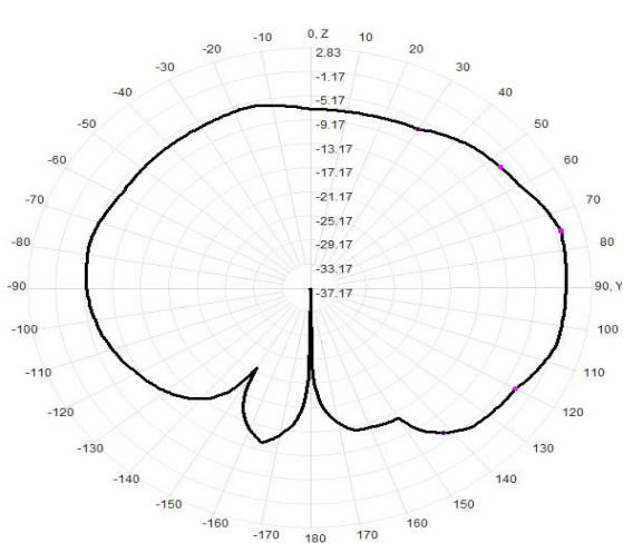
870.0MHz Total(E2-YZ)
