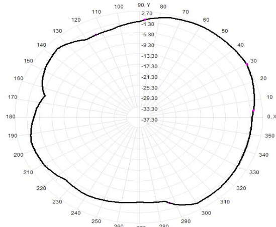
870.0MHz Total(E1-XZ)
