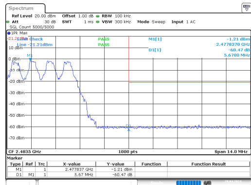
GFSK_Hopping_Upper
