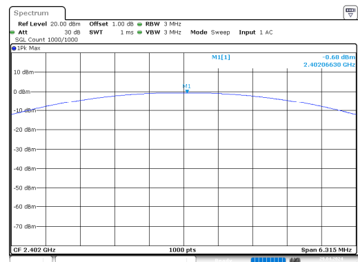
\pi/4 -DQPSK_Low
