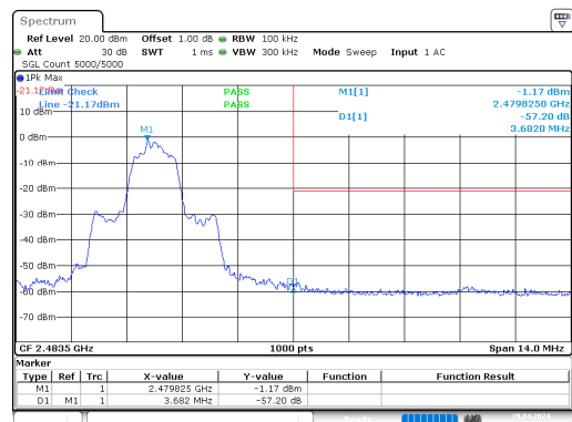
\pi/4 -DQPSK_High
