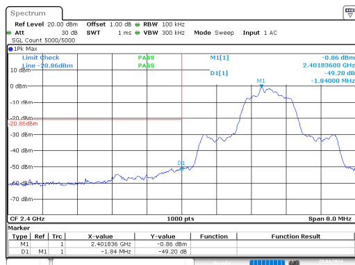
\pi/4 -DQPSK_Low
