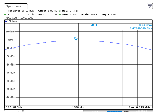
\pi/4 -DQPSK_High
