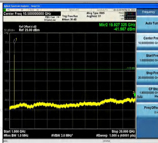
Band4-1413-4-1000~20000MHz-PASS
