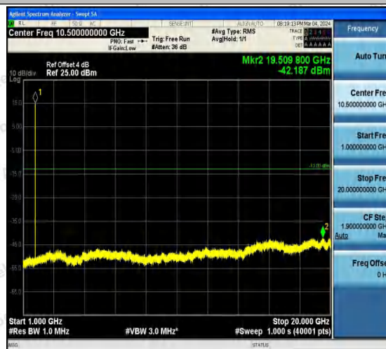
Band4-1513-5-1000~20000MHz-PASS
