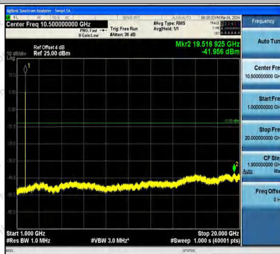
Band4-1413-5-1000~20000MHz-PASS
