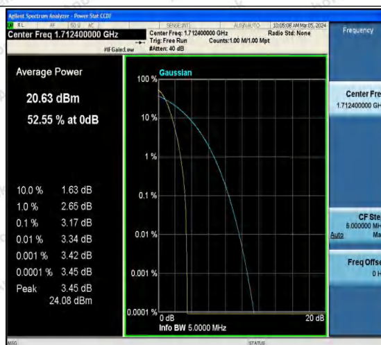
Band4-1312-1-PASS
