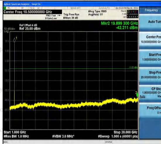
Band4-1312-4-1000~20000MHz-PASS
