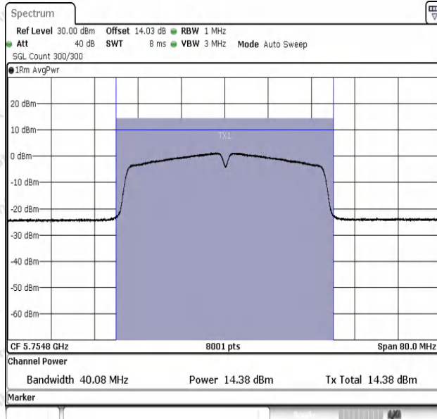
11N40SISO-Ant1-5755-PASS
