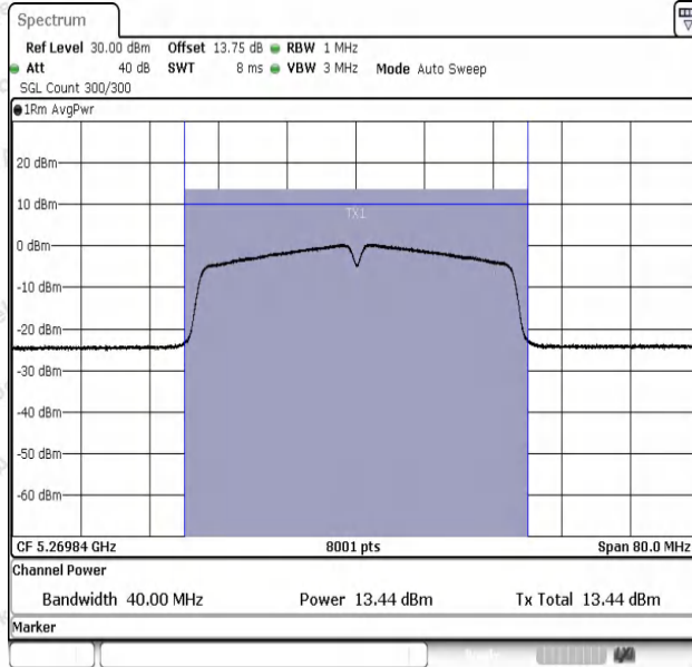
11N40SISO-Ant1-5270-PASS
