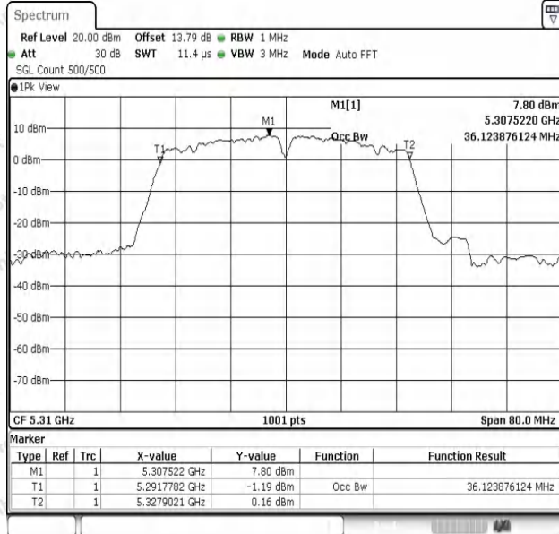
11N40SISO-Ant1-5310
