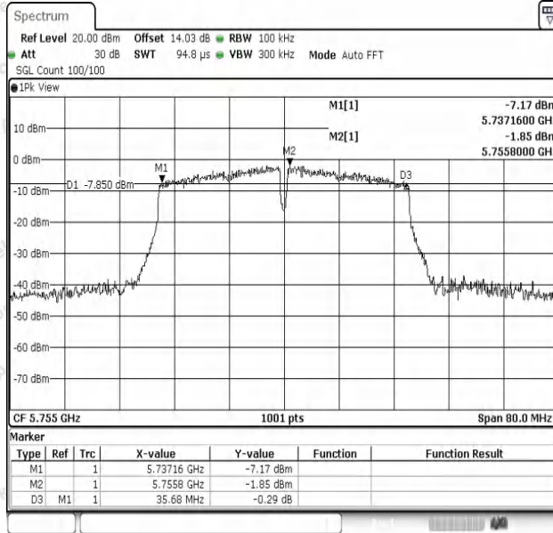
11N40SISO-Ant1-5755-PASS
