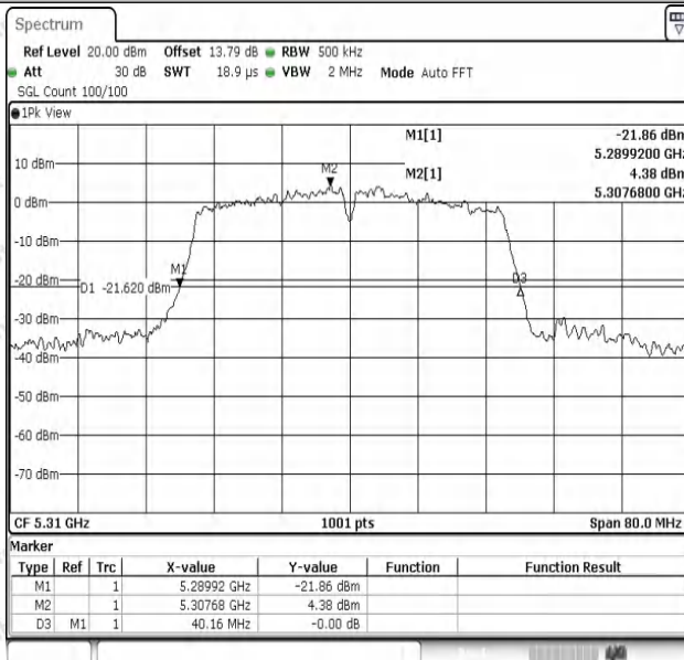
11N40SISO-Ant1-5310
