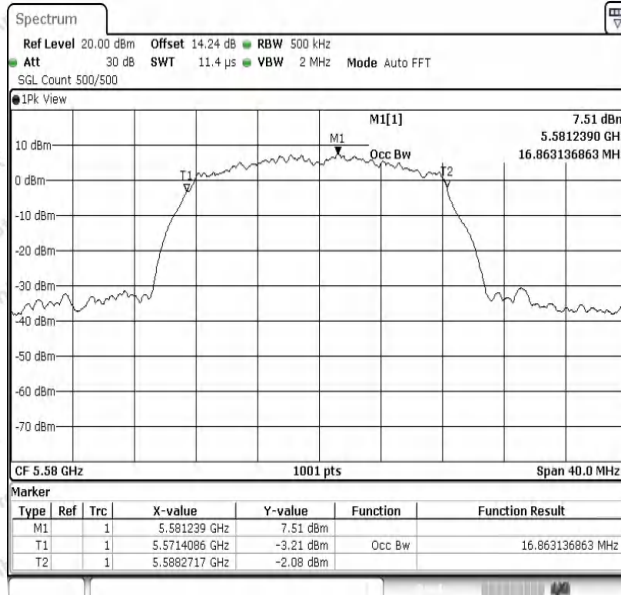
11A-Ant1-5580
