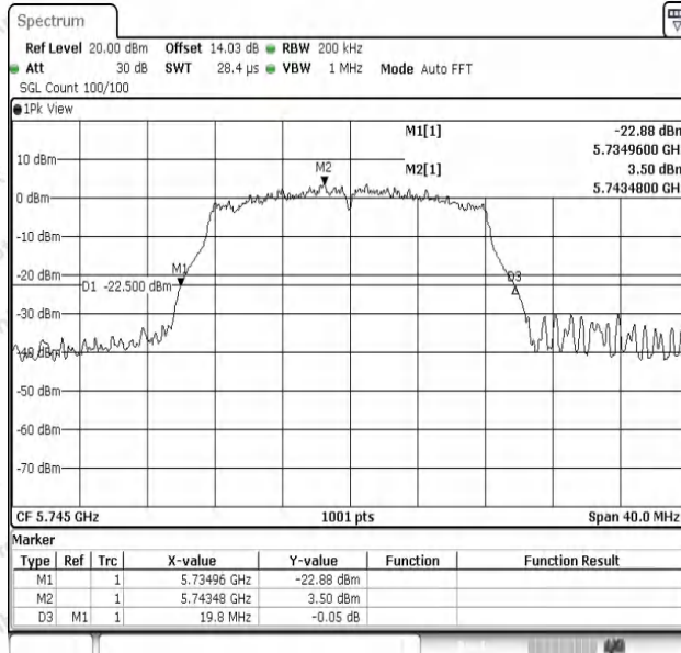
11A-Ant1-5745
