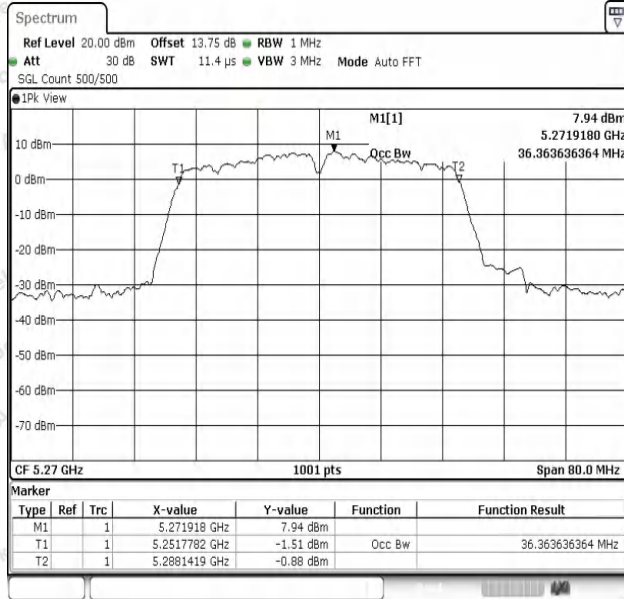
11N40SISO-Ant1-5270
