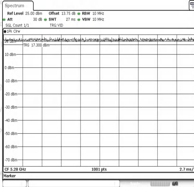
NTNV-11A-Ant1-5280
