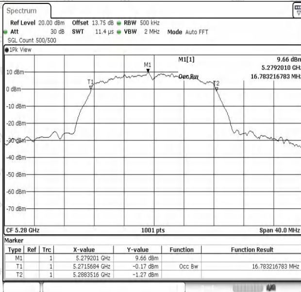
11A-Ant1-5280
