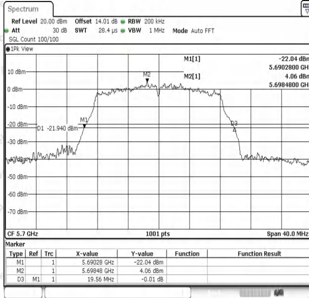
11A-Ant1-5700
