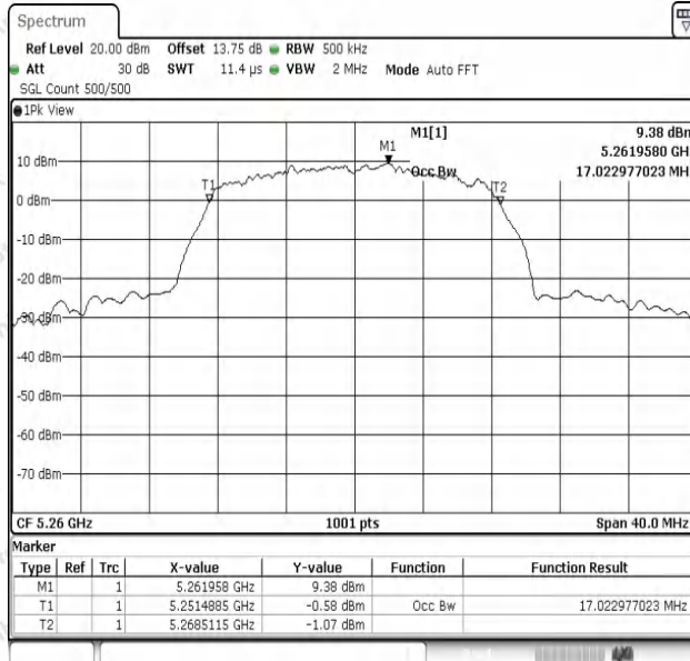
11A-Ant1-5260
