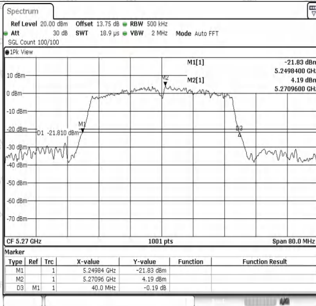
11N40SISO-Ant1-5270
