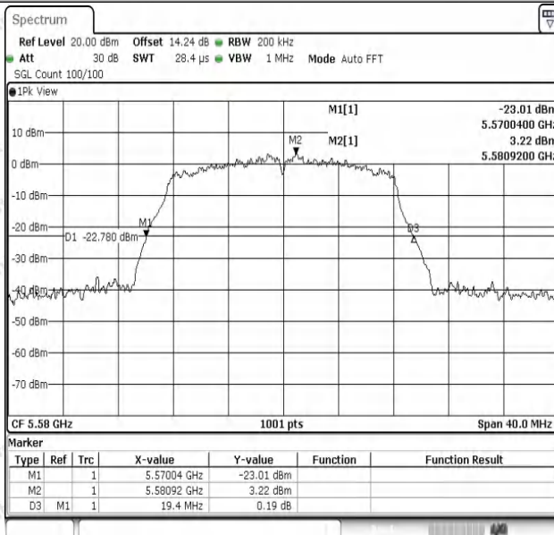
11A-Ant1-5580
