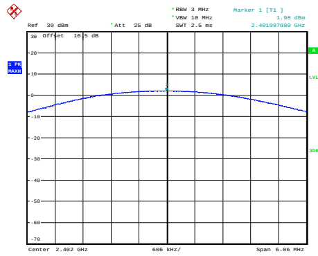
\pi/4 -DQPSK_Low_2DH1
