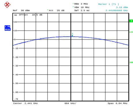
\pi/4 -DQPSK_Mid_2DH1
