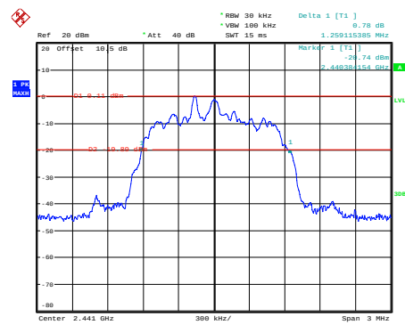
\pi/4 -DQPSK_Mid_2DH1
