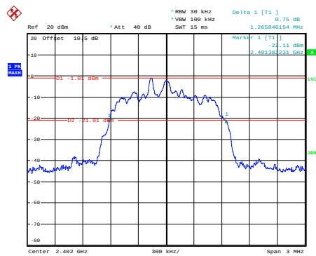
\pi/4 -DQPSK_Low_2DH1
