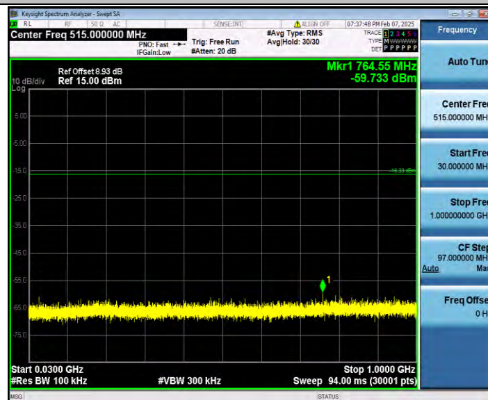
11AX20SISO_Ant0_2412_30~1000
