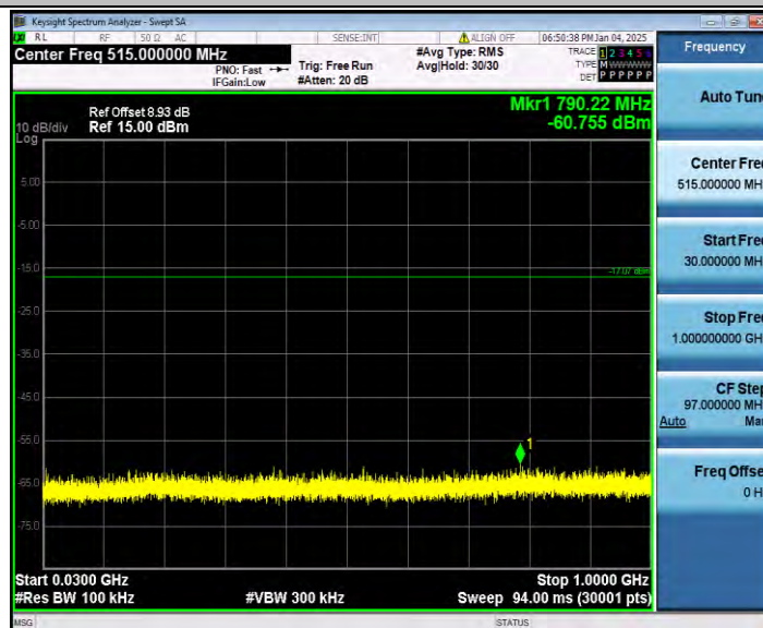
11N20ISO_Ant0_2412_30~1000
