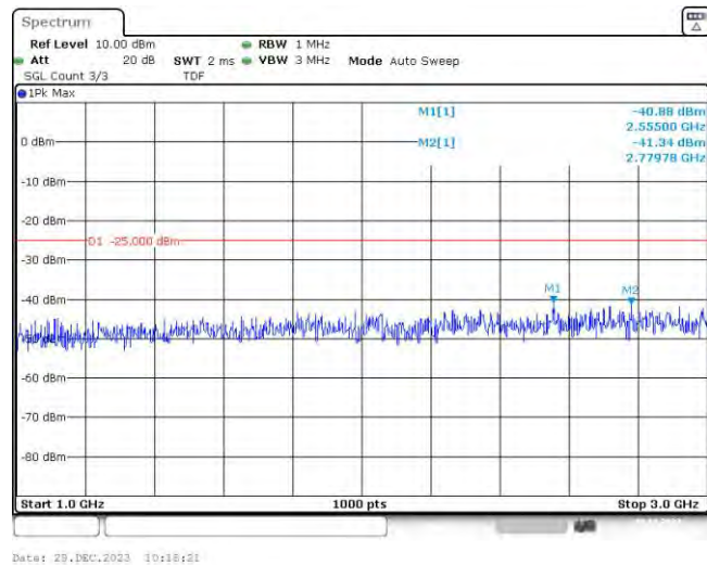
Band41-5MHz-QPSK-40265-25RB#0-Range2:1000~3000MHz
