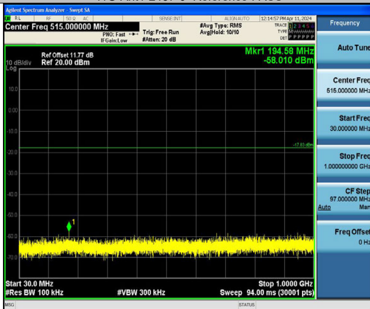
11G-Ant1-2437-30~1000-PASS
