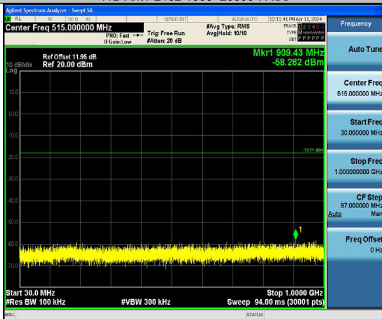
11G-Ant1-2412-30~1000-PASS
