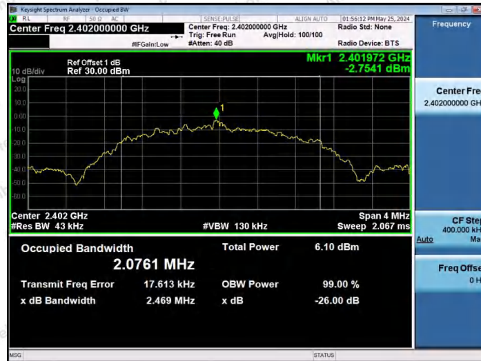
BLE_2M-Ant1-2402
