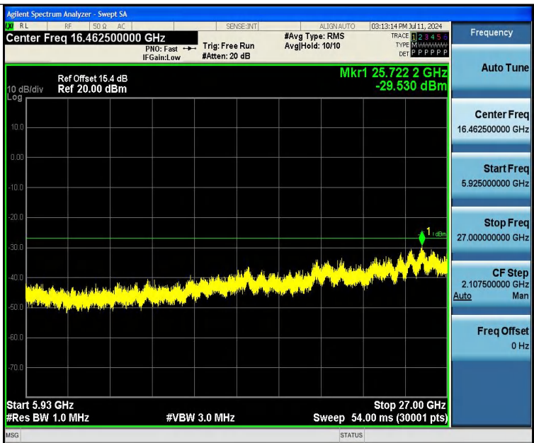
11AC80SISO-Ant1-5775-5925~40000-PASS
