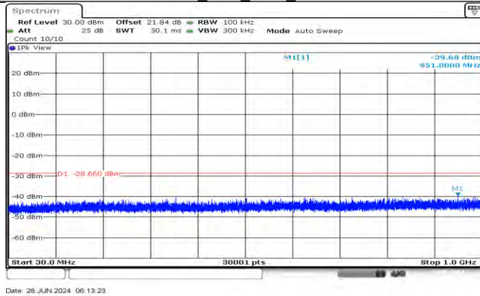
11AX40SISO_Ant1_2452_30~1000
