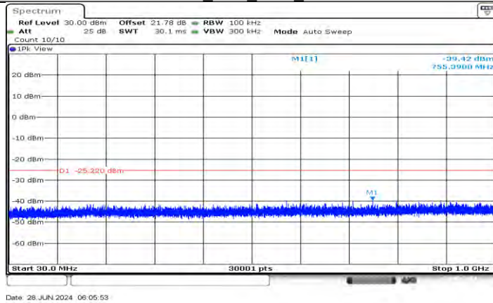
11AX20SISO_Ant1_2412_30~1000
