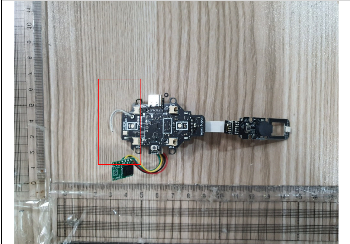
ANTENNA(2.4 GHz)
