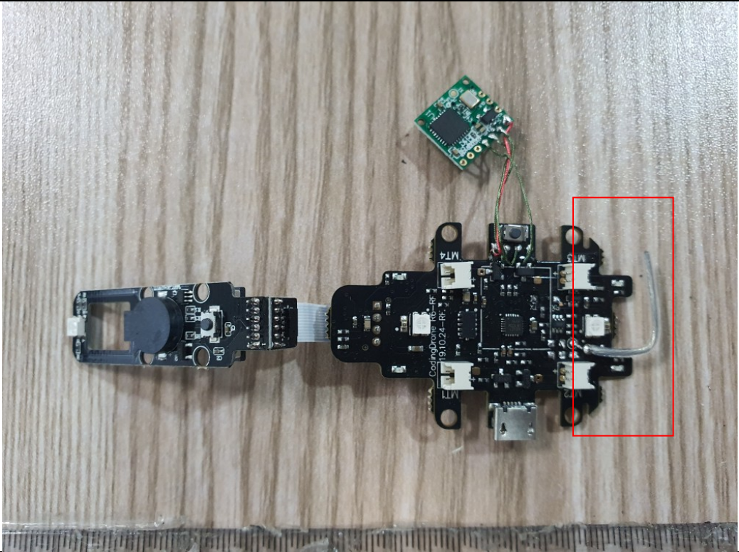
ANTENNA(2.4 GHz)
