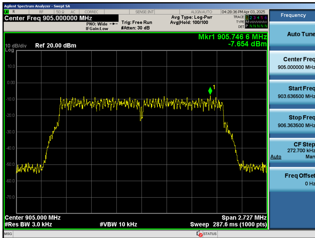
Test_Graph_802.11ah_ANT1_905_BW 2MHz_ PSD
