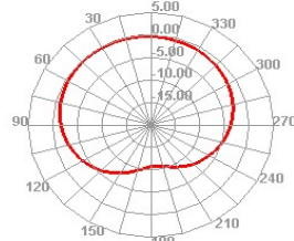
902.000MHz H
