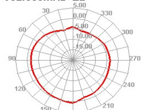
902.000MHz E2
