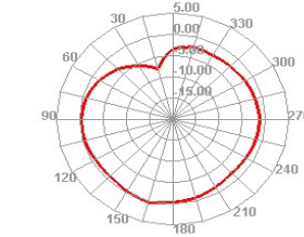
920.000MHz E2
