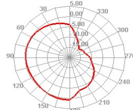
902.000MHz E1
