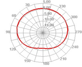
920.000MHz H
