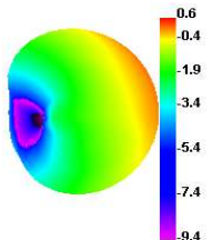
920.000MHz
