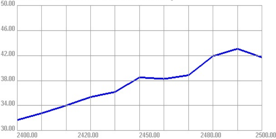
2400.00MHz - 2500.00MHz Efficiency
