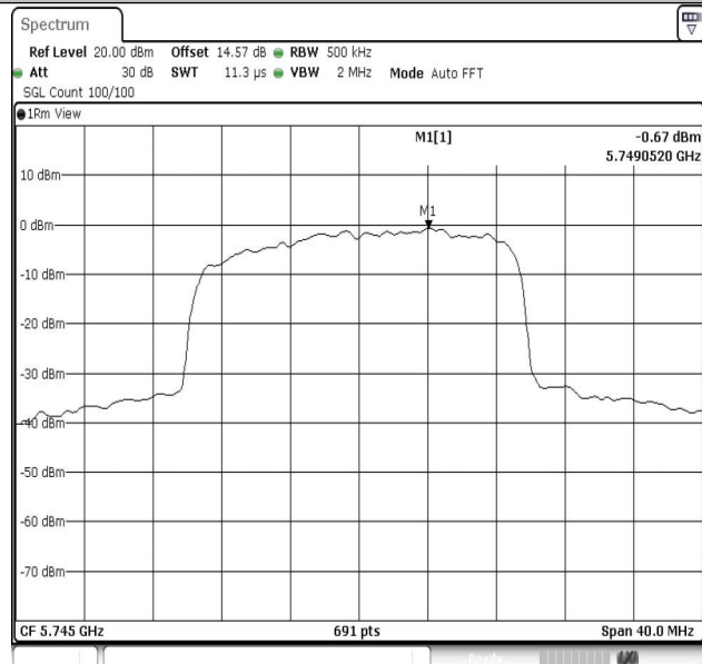
11AX20MIMO-Ant1-5745-PASS
