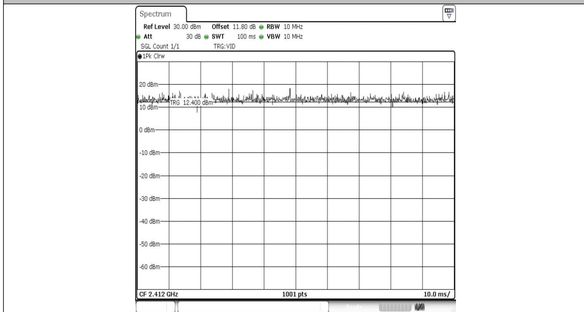
NTNV-11AX20MIMO-Ant1-2412
