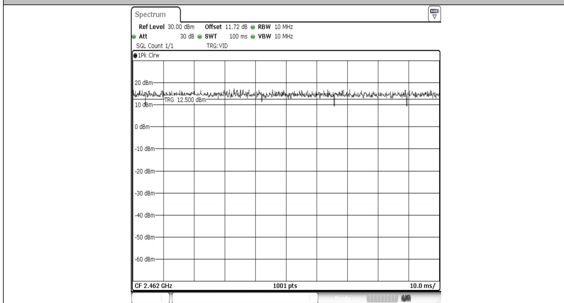
NTNV-11AX20MIMO-Ant1-2462
