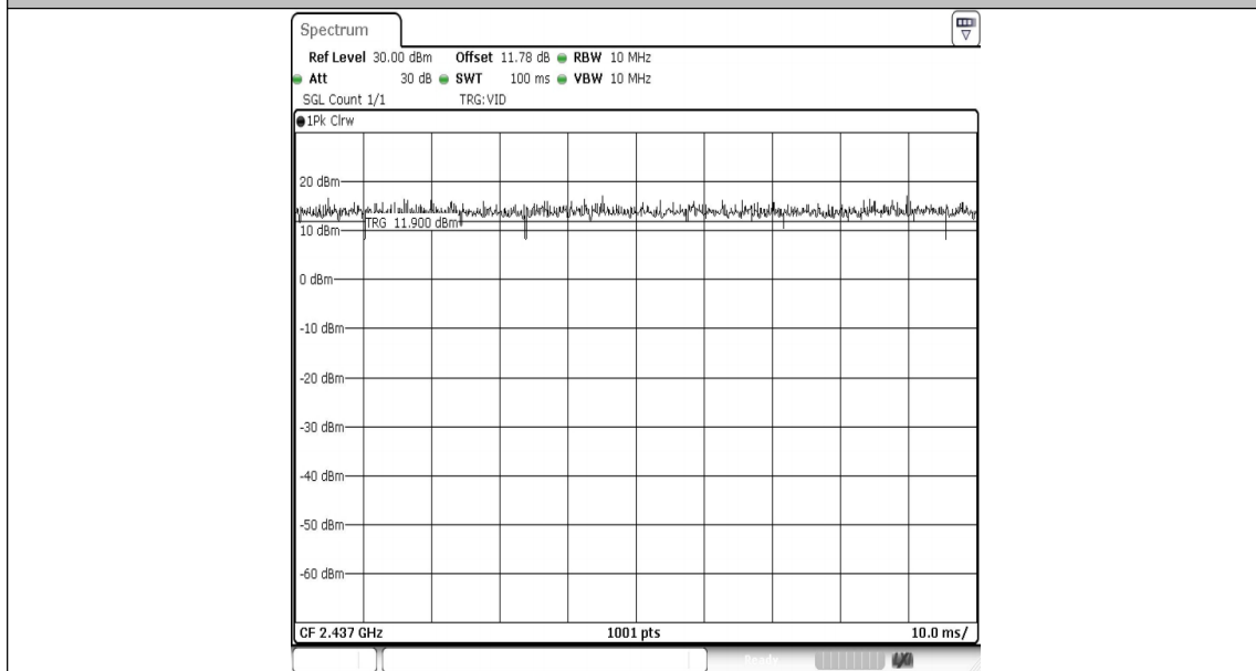
NTNV-11AX20MIMO-Ant1-2437
