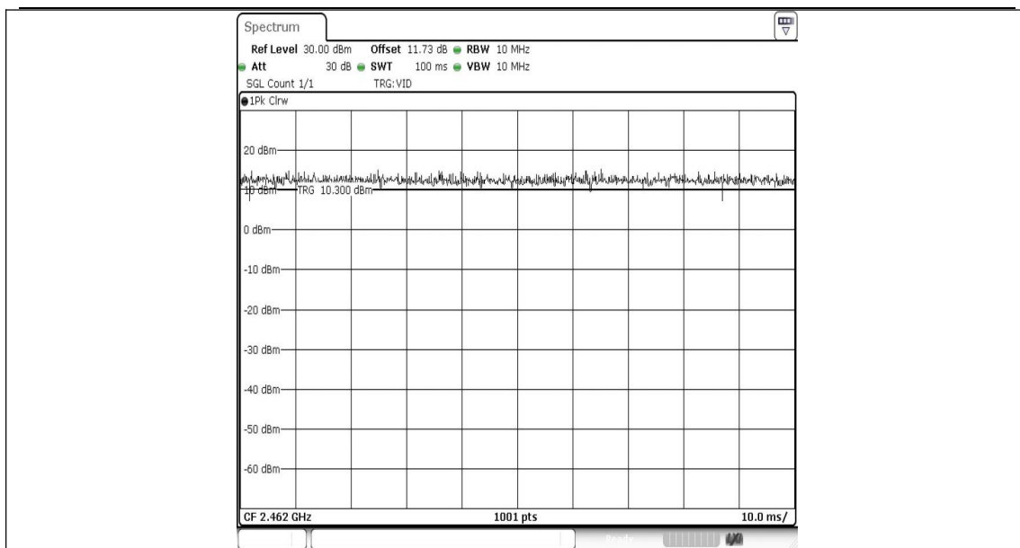
NTNV-11AX20MIMO-Ant1-2462
