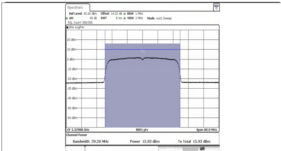
11AX40MIMO-Ant1-5230-PASS
