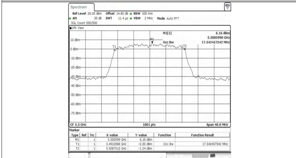
11N20MIMO-Ant1-5500
