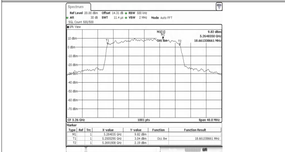
11AX20MIMO-Ant1-5260
