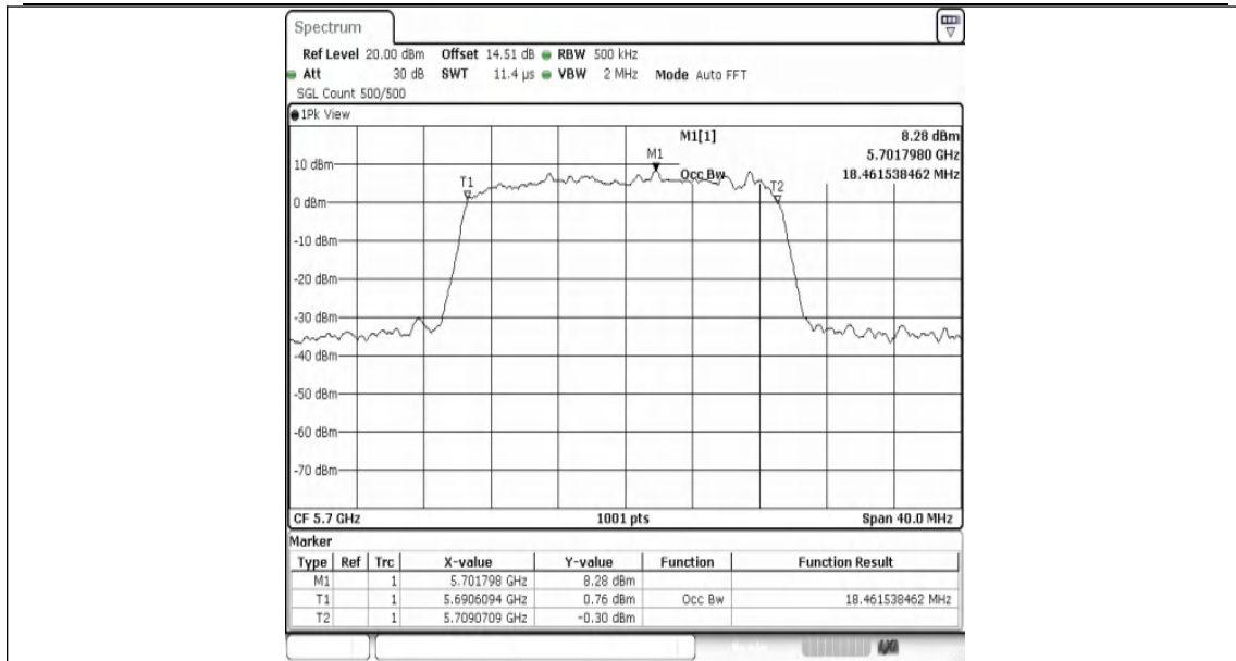
11AX20MIMO-Ant1-5700
