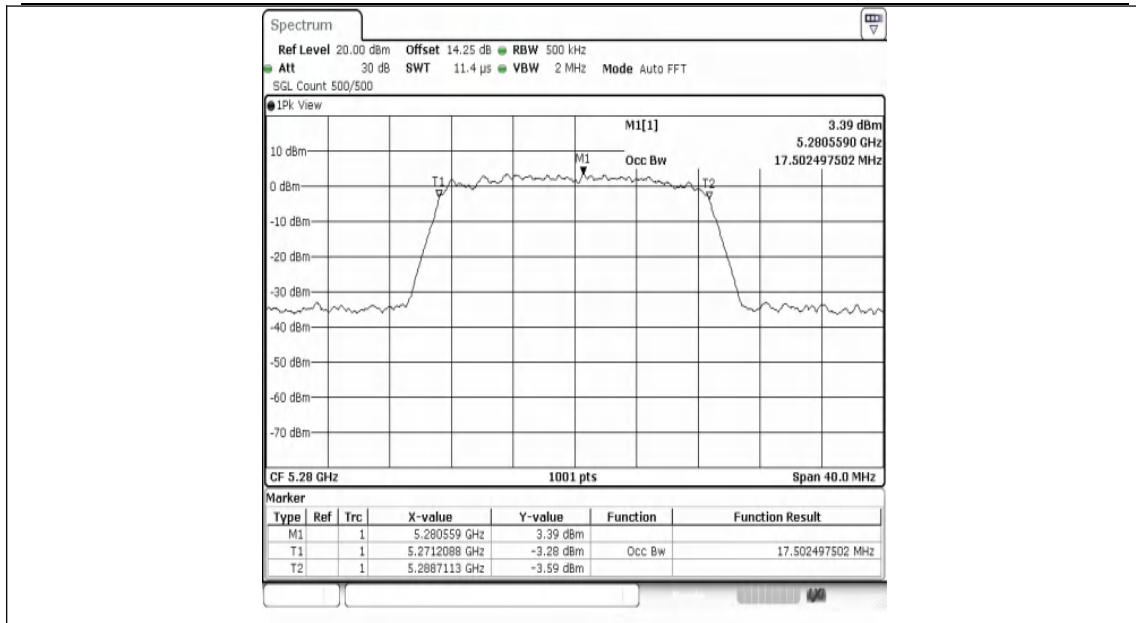
11AC20MIMO-Ant1-5280
