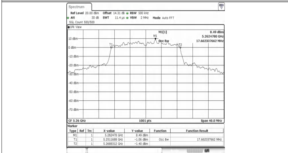
11AC20MIMO-Ant1-5260
