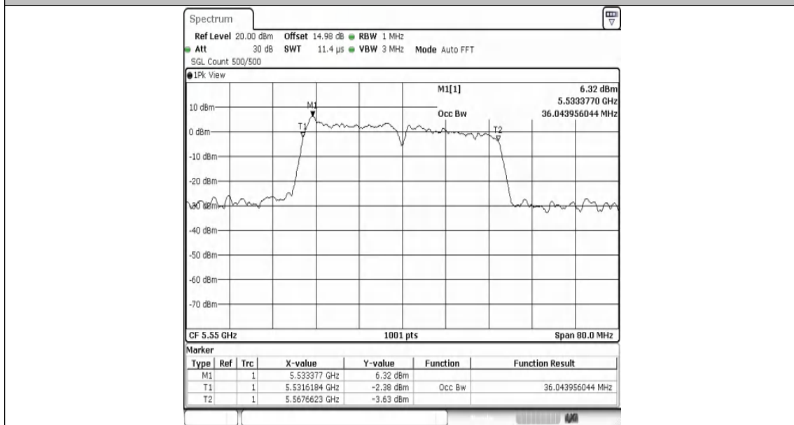
11N40MIMO-Ant1-5550
