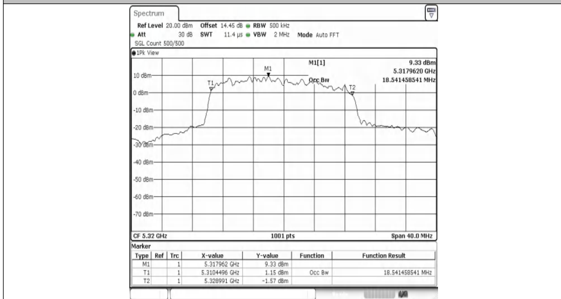
11AX20MIMO-Ant1-5320
