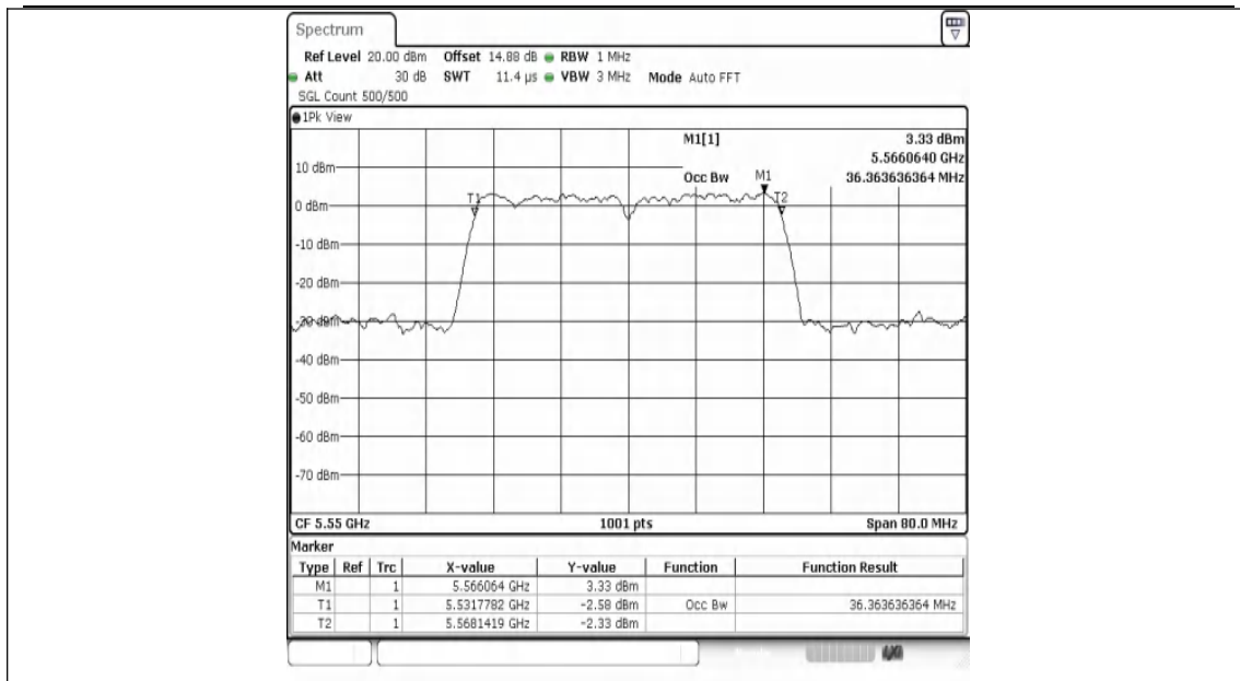
11N40MIMO-Ant1-5550
