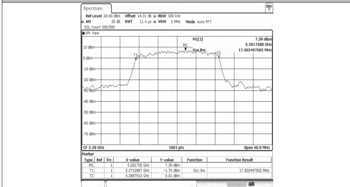
11AC20MIMO-Ant1-5280
