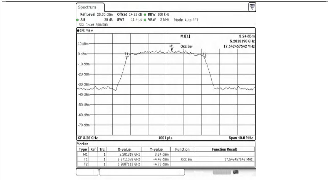
11N20MIMO-Ant1-5280
