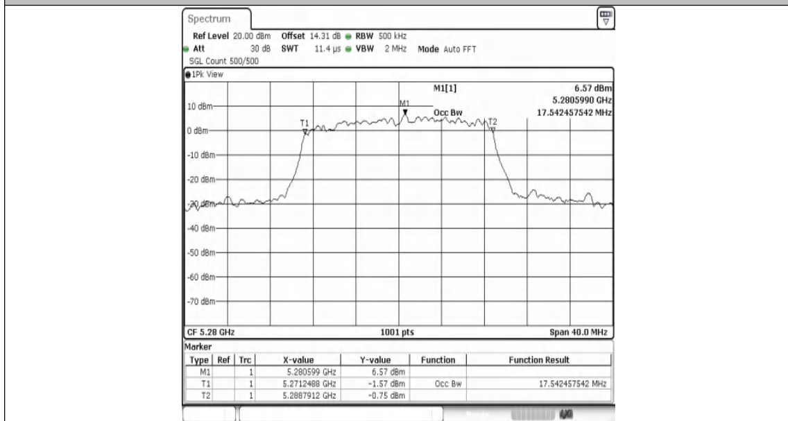
11N20MIMO-Ant1-5280
