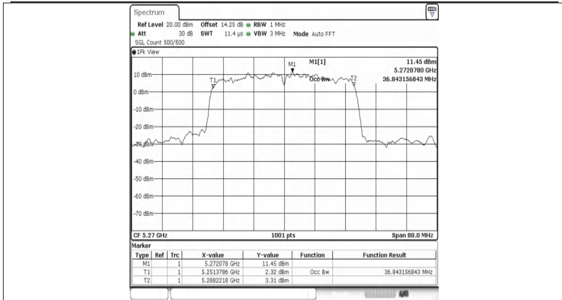
11AX40MIMO-Ant1-5270
