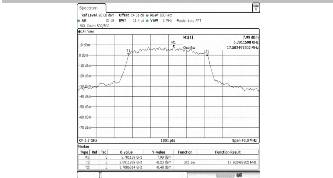
11N20MIMO-Ant1-5700
