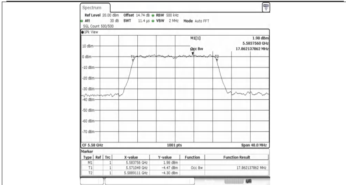
11N20MIMO-Ant1-5580
