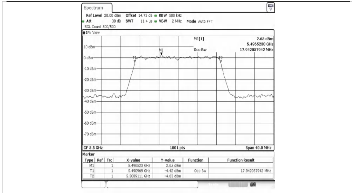
11N20MIMO-Ant1-5500
