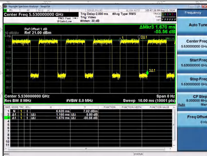
NTNV-11AC80SISO-Ant1-5530
