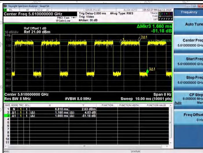
NTNV-11AC80SISO-Ant1-5610
