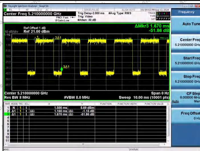
NTNV-11AC80SISO-Ant1-5210
