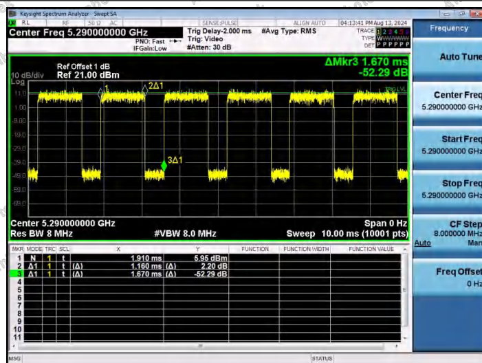
NTNV-11AC80SISO-Ant1-5290
