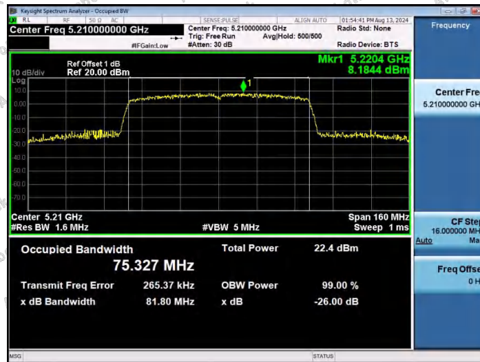
11AC80SISO-Ant1-5210
