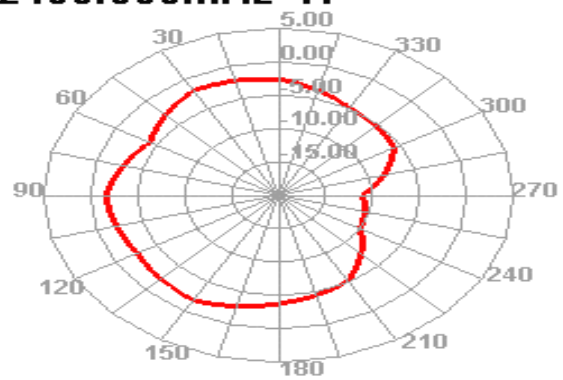
2400.000MHz H
