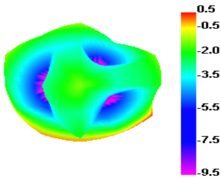
2400.000MHz E1
