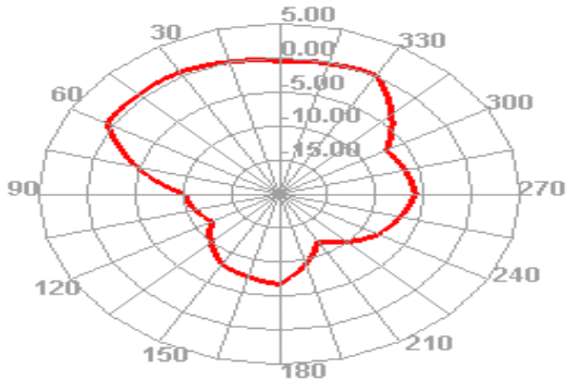
2500.000MHz E1
