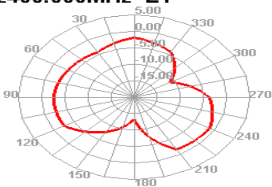
2400.000MHz E1
