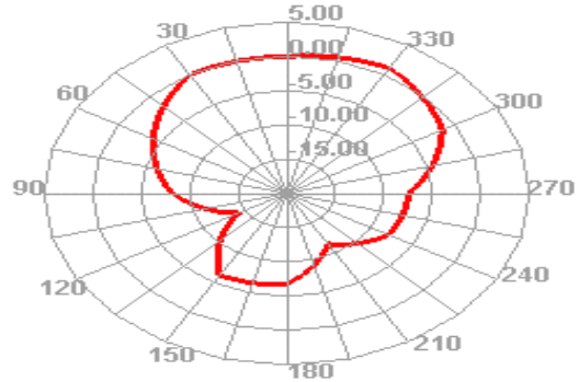
2500.000MHz E2
