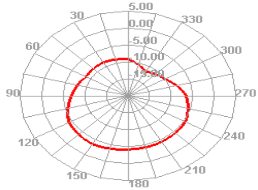
2450.000MHz H
