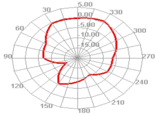
2450.000MHz E2
