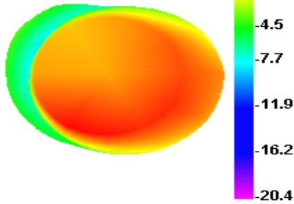
2450.000MHz E1
