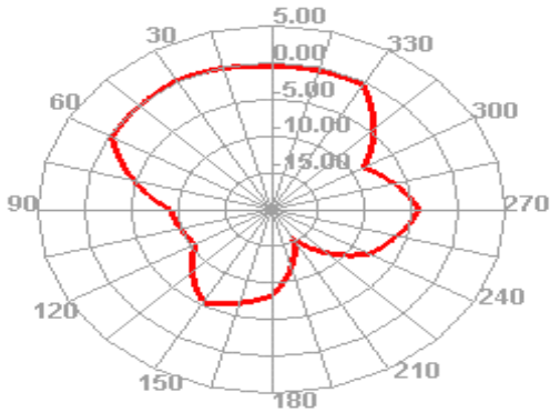
2450.000MHz E1
