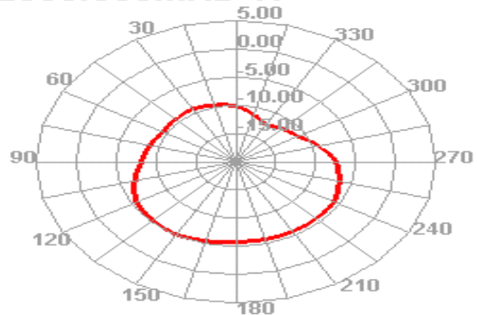
2500.000MHz H
