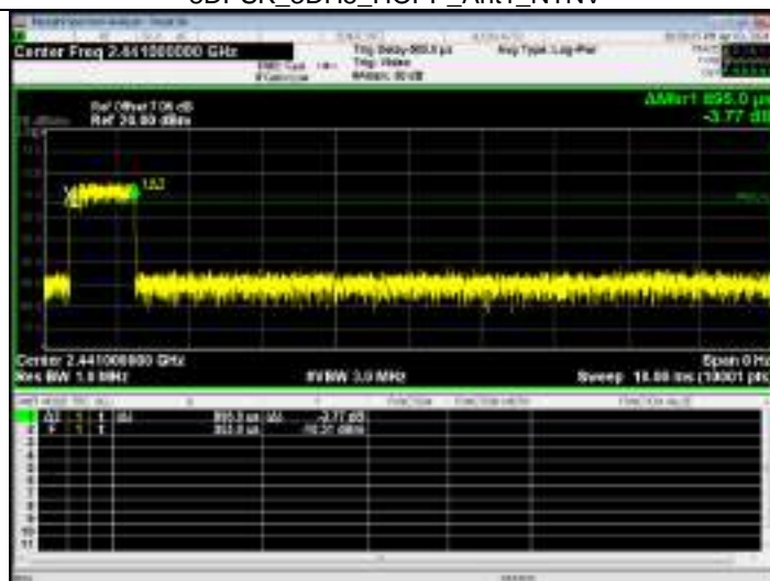
8DPSK_3DH5_HOPP_Ant1_NTNV
