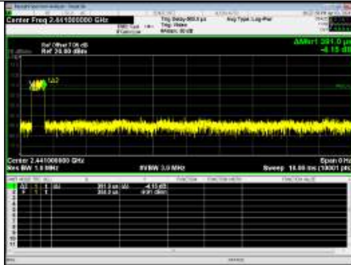
Pi/4DQPSK_2DH3_HOPP_Ant1_NTNV
